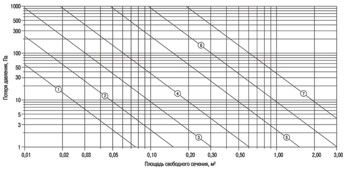
Зависимость падения давления от площади свободного сечения решетки ВР-НЗ, ВР-Н4
